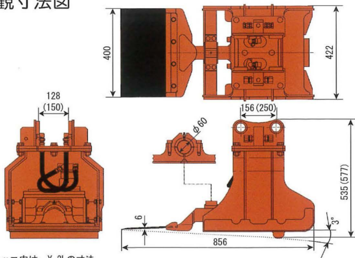
外観寸法図
